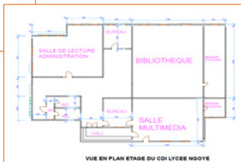
VUE EN PLAN ETAGE DU CDI LYCEE NGOYE
